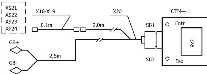
3.4. Монтажная схема СТМ-4.1
