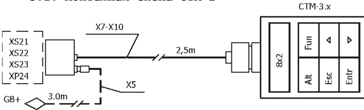
3.2. Монтажная схема СТМ-3.х и СТМ-5
